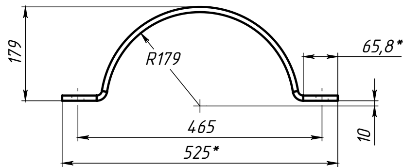
Поз.4 (Полухомут)
